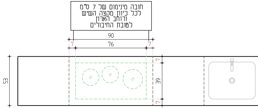
מבט עליון לדוגמה 3 מוקדי בישול
