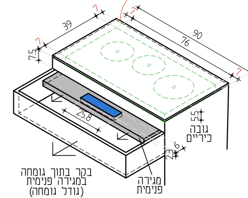
חובה מינימום של 7 ס"מ לכל כיוון מקצה השיש ורוחב הארון לשורת החיבורים
